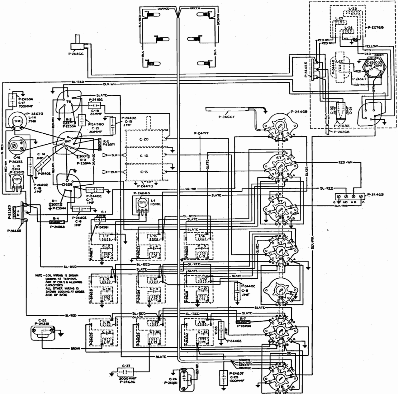
Fig. 3. Wiring Diagram.
