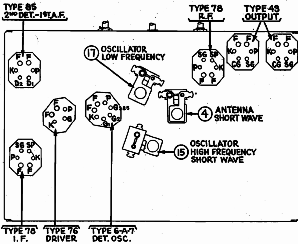
Fig. 1—Tube Sockets
