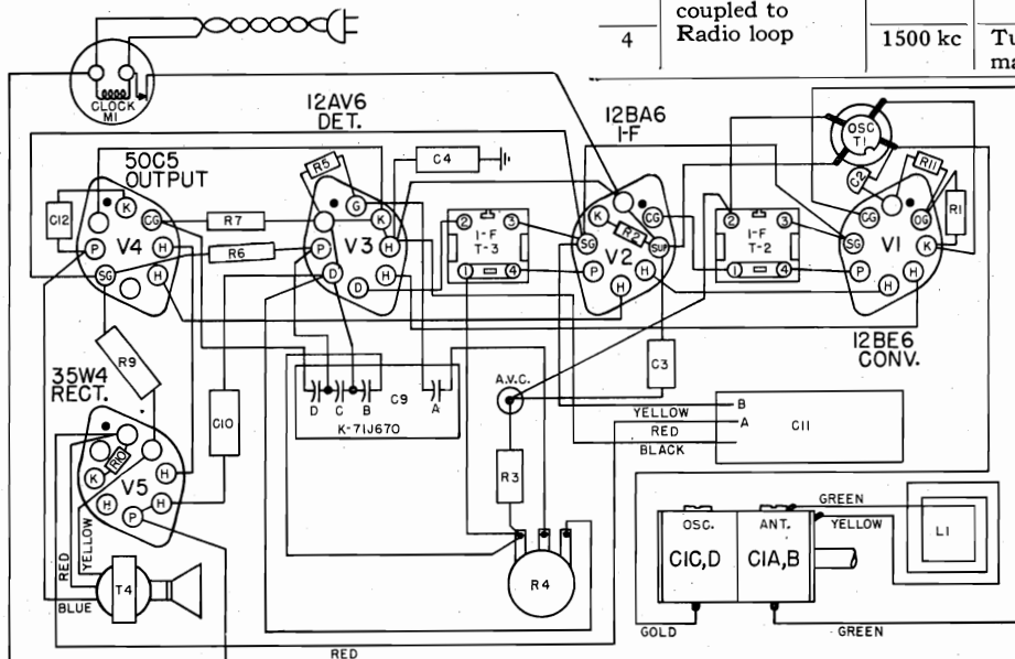
Fig. 7. Wiring Diagram
