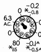
6SQ7GT A.F.—(A-M) DET.—A.V.C.
